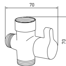
M22 x 1
