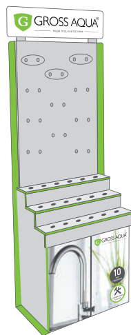
СТЕНД ПОД СМЕСИТЕЛИ Размер: 2300 × 850 × 470 мм Вмещает 29 смесителей: 11 настенных и 18 настольных
