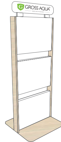
СТЕНД ПОД АКСЕССУАРЫ ДЛЯ ВАННОЙ Размер: 1900 × 732 × 700 мм Вмещает 38 видов аксессуаров для ванной
